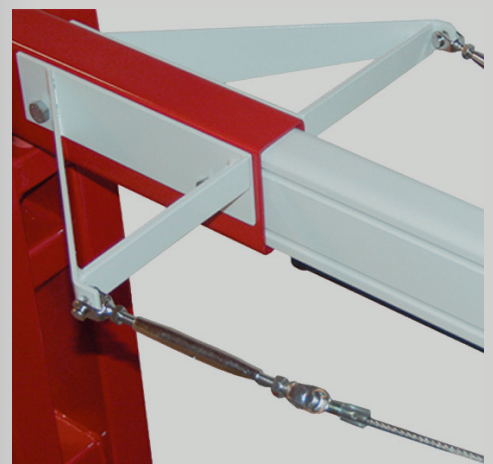
Abspannung ab EH 55L
